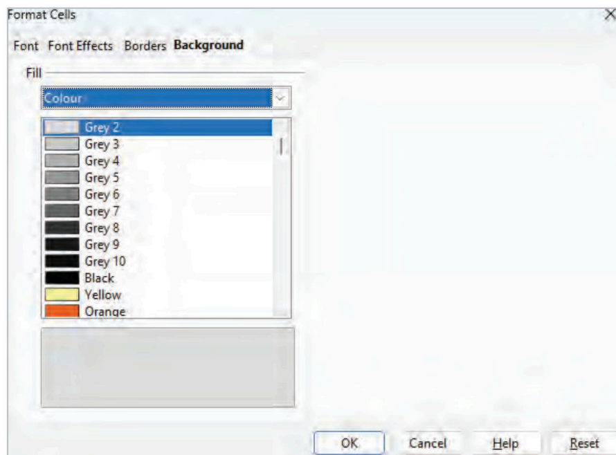
Fig. 19.12: Table Background
